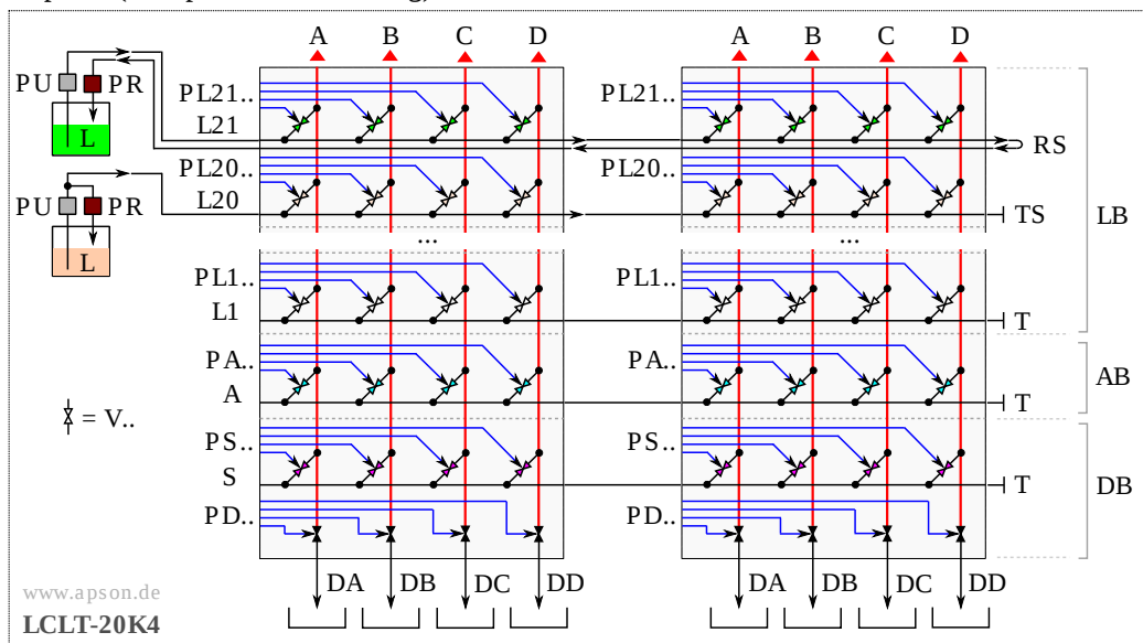
Abb. 2: APSON LCLT-20K4 -- Funktionsschema (für 2 Lackwechsler)
