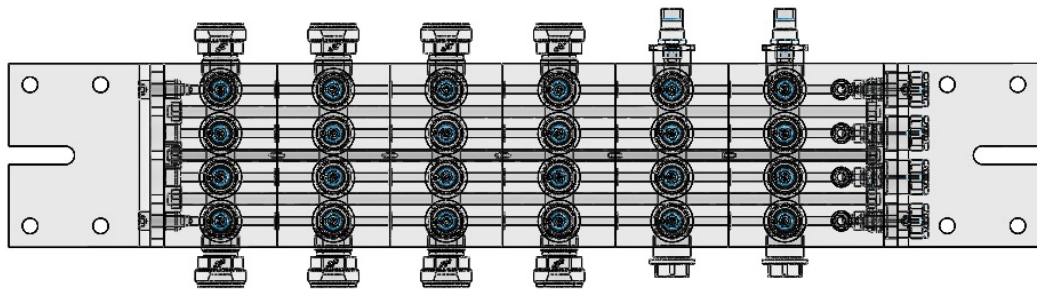
Abb. 1: APSON LCLT-20K4 Inline für 4 Lacke (mit 1 Luft- und 1 Dumpblock)
